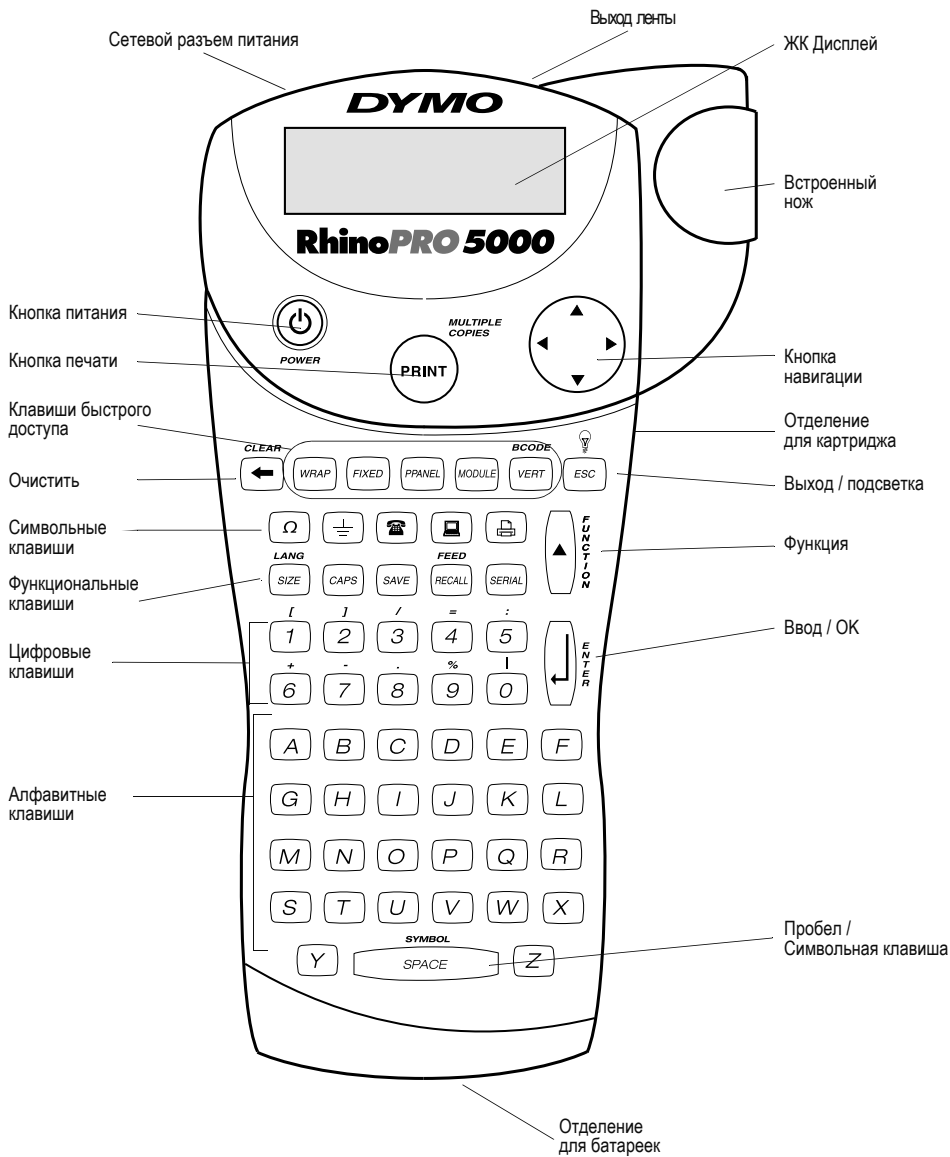
Рисунок 1 Принтер RhinoPRO 5000
